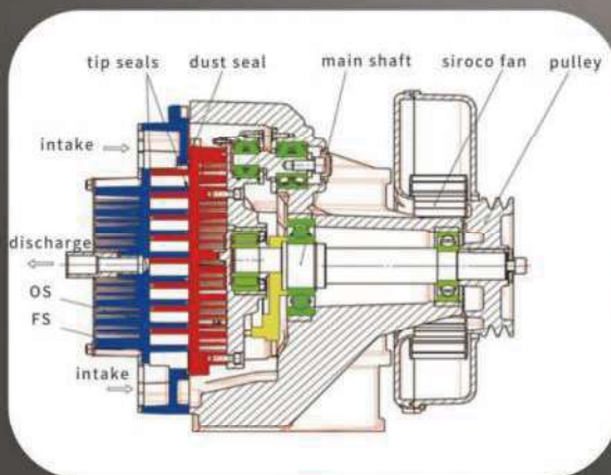
皮帶傳動式
